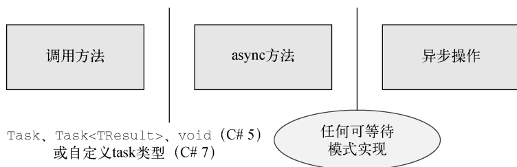
图 5-4 可等待模式允许 async 方法异步地等待操作执行完成
