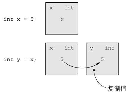
图 13-2 把值赋给一个新变量
