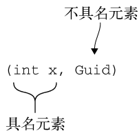
图 11-2 包含元素类型为 int 和 Guid 的元组类型，第 1 个类型的名称为 x
