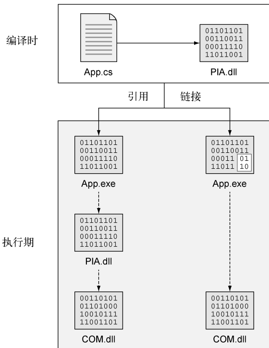
图 4-3 引用与链接的对比
