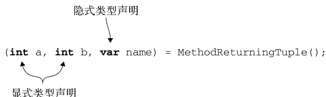
图 12-1 在分解操作中混用显式类型和隐式类型
