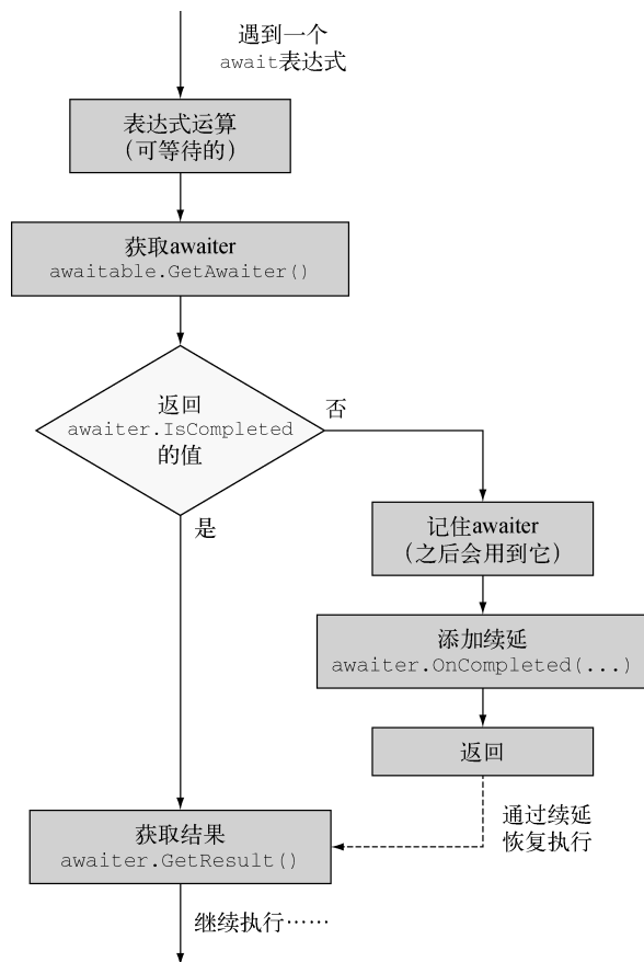
图 5-7 通过可等待模式处理 await
