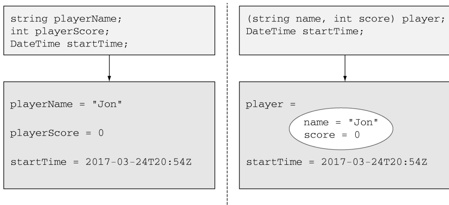
图 11-3 左边三个独立变量，右边两个变量，其中一个是元组
