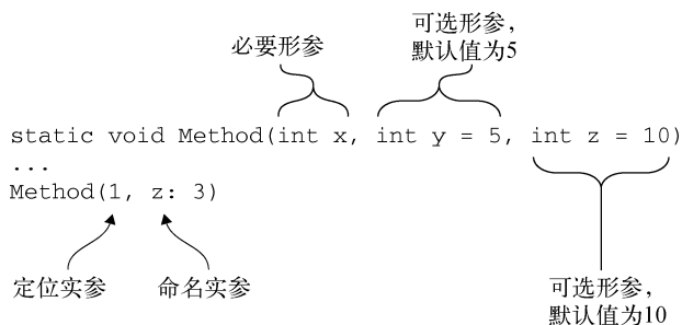
图 4-2 可选形参/必要形参与命名实参/定位实参的语法
