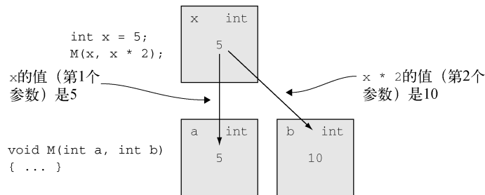
图 13-3 使用值参数调用方法：方法形参是新变量，其初始值是实参的值
