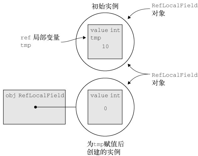
图 13-6 在代码清单 13-4 末尾，tmp 变量指向第一个实例创建后的字段，而 obj 指向另外一个实例
