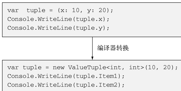
图 11-5 编译器把元素类型替换成 ValueTuple
