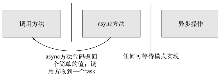
图 5-5 async 方法返回值给调用方
