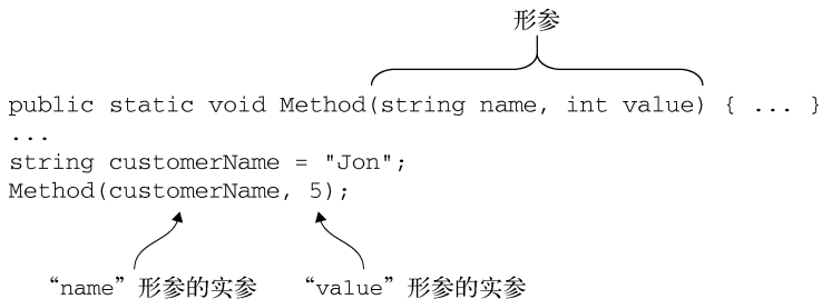
图 2-1 函数形参与实参的关系
