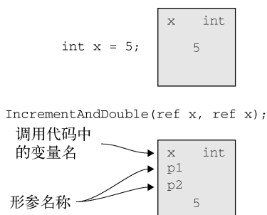
图 13-5 两个 ref 参数指向同一张纸
