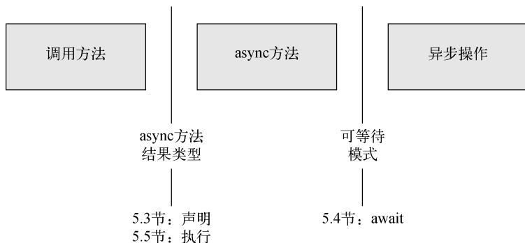
图 5-3 5.3 节、5.4 节和 5.5 节内容在理论模型中的位置
