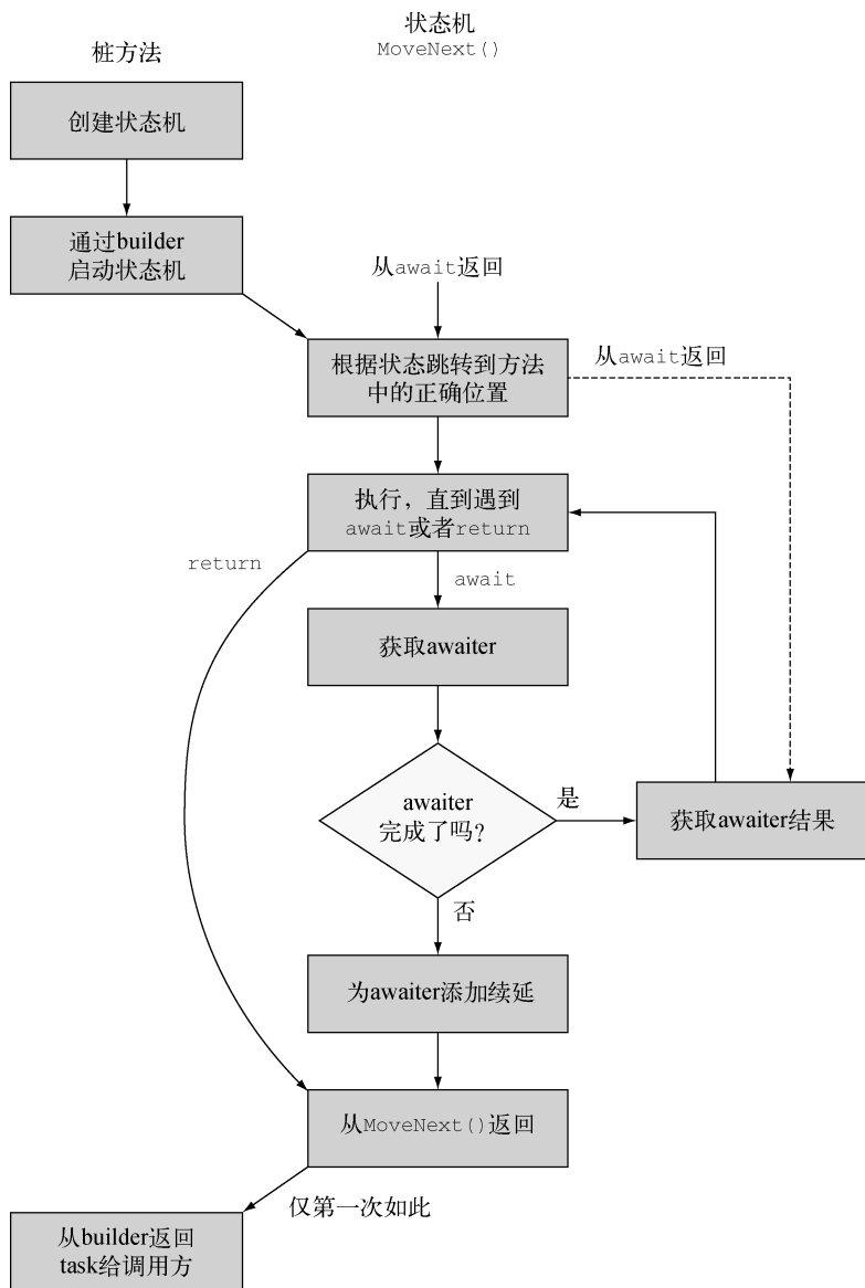
图 6-2 async 方法流程图
