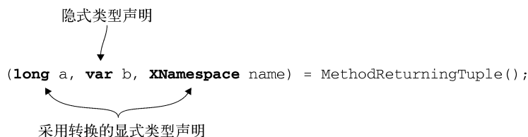
图 12-2 包含隐式转换的分解操作
