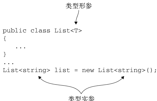
图 2-2 类型形参与类型实参之间的关系
