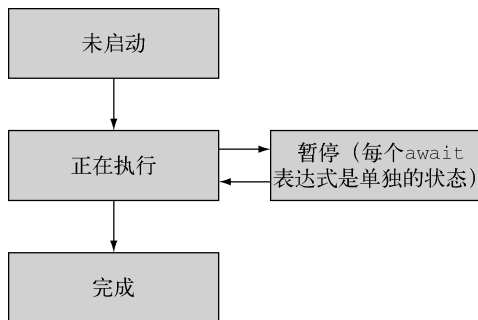
图 6-1 状态之间的转换
