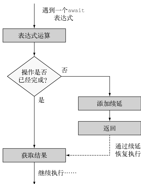
图 5-6 await 处理流程图
