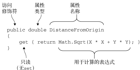
图 8-1 标注了重点的属性声明
