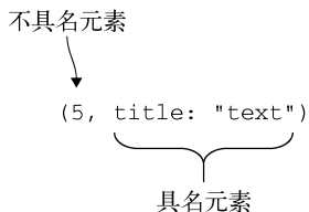
图 11-1 包含元素值为 5 和 "text" 的元组字面量，第 2 个元素的名称为 title
