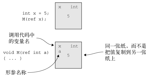
图 13-4 ref 参数使用同一张纸，而不是创建一张新纸并复制值
