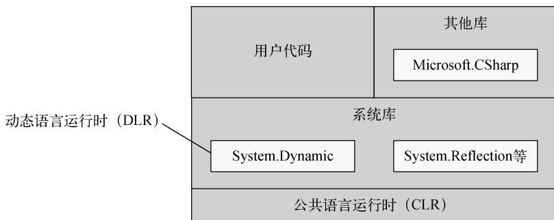
图 4-1 动态类型所涉组件图示
