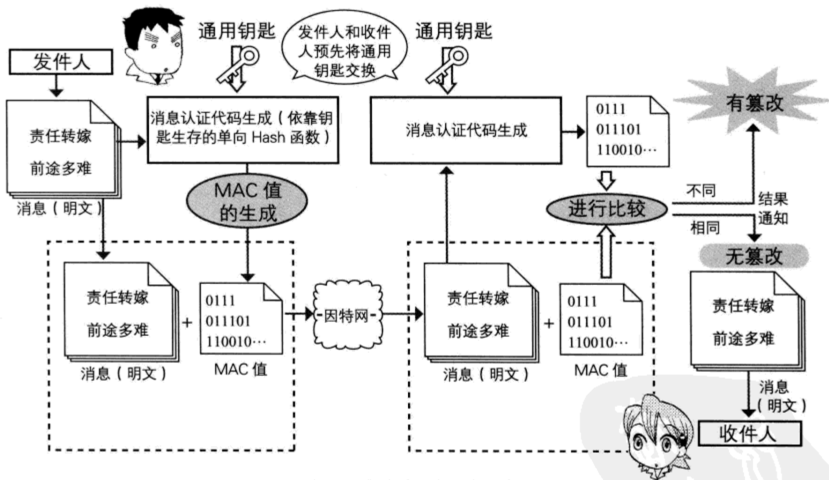
图 4.3 消息认证代码的构成
