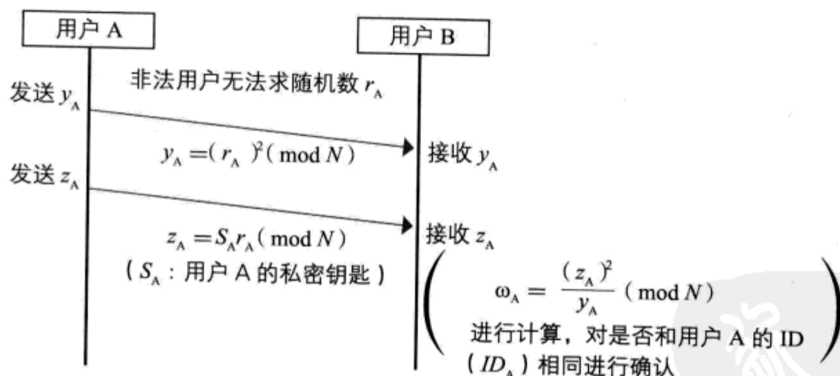
图 4.10 对于零知识对话证明 (真实性) 的确认程序
