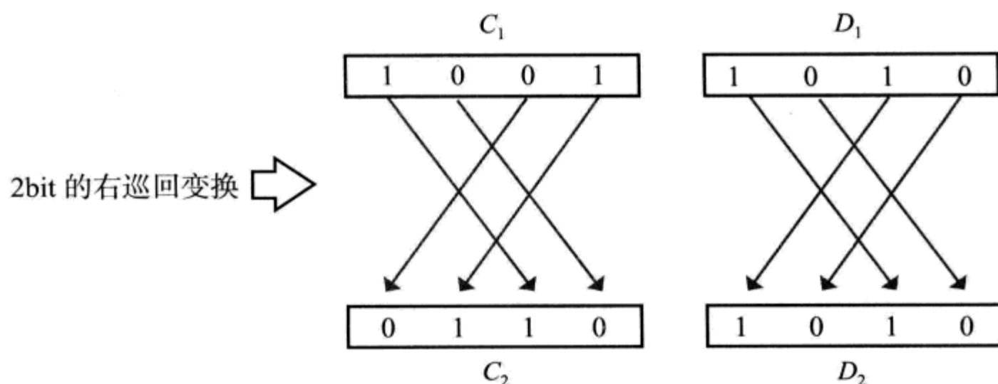
图 2.33 右巡回变换的处理 (步骤 4)
