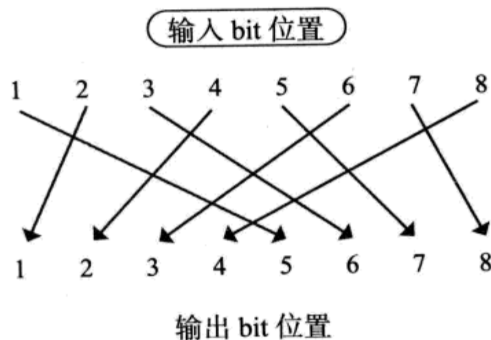
图 2.13 初期置换 IP
