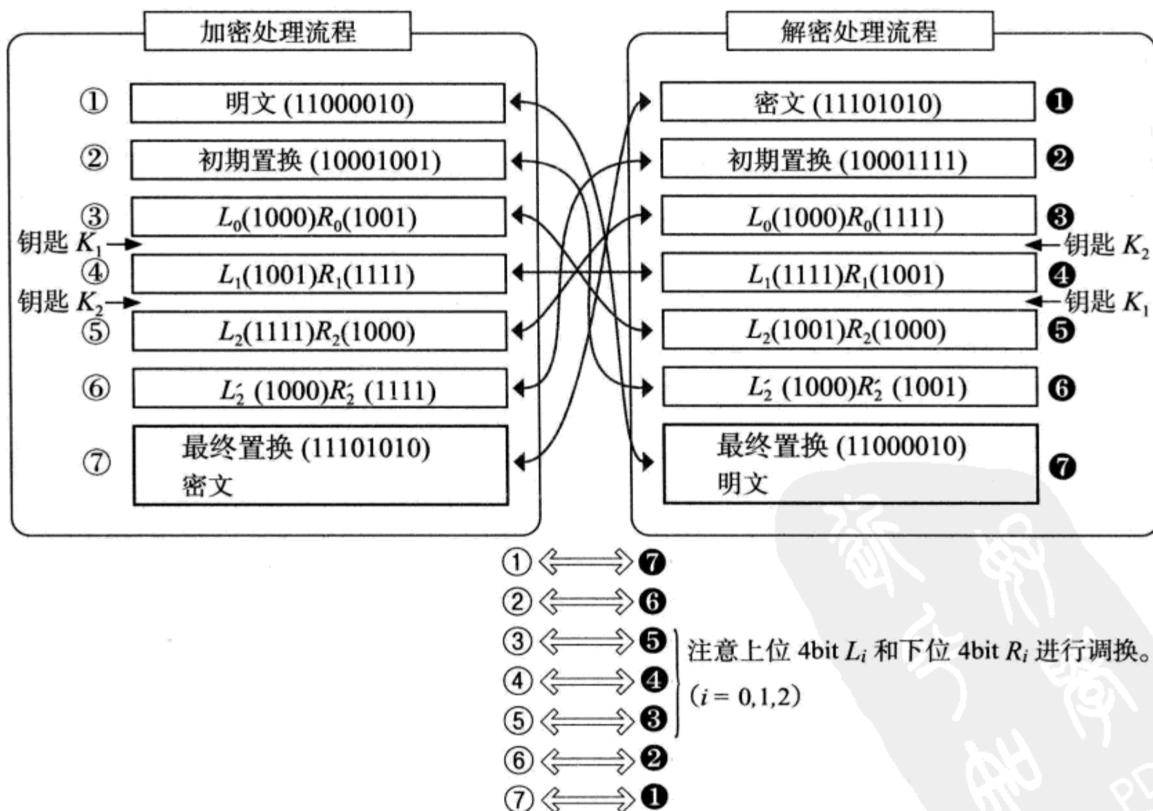
图 2.24 加密处理和解密处理的对应关系
