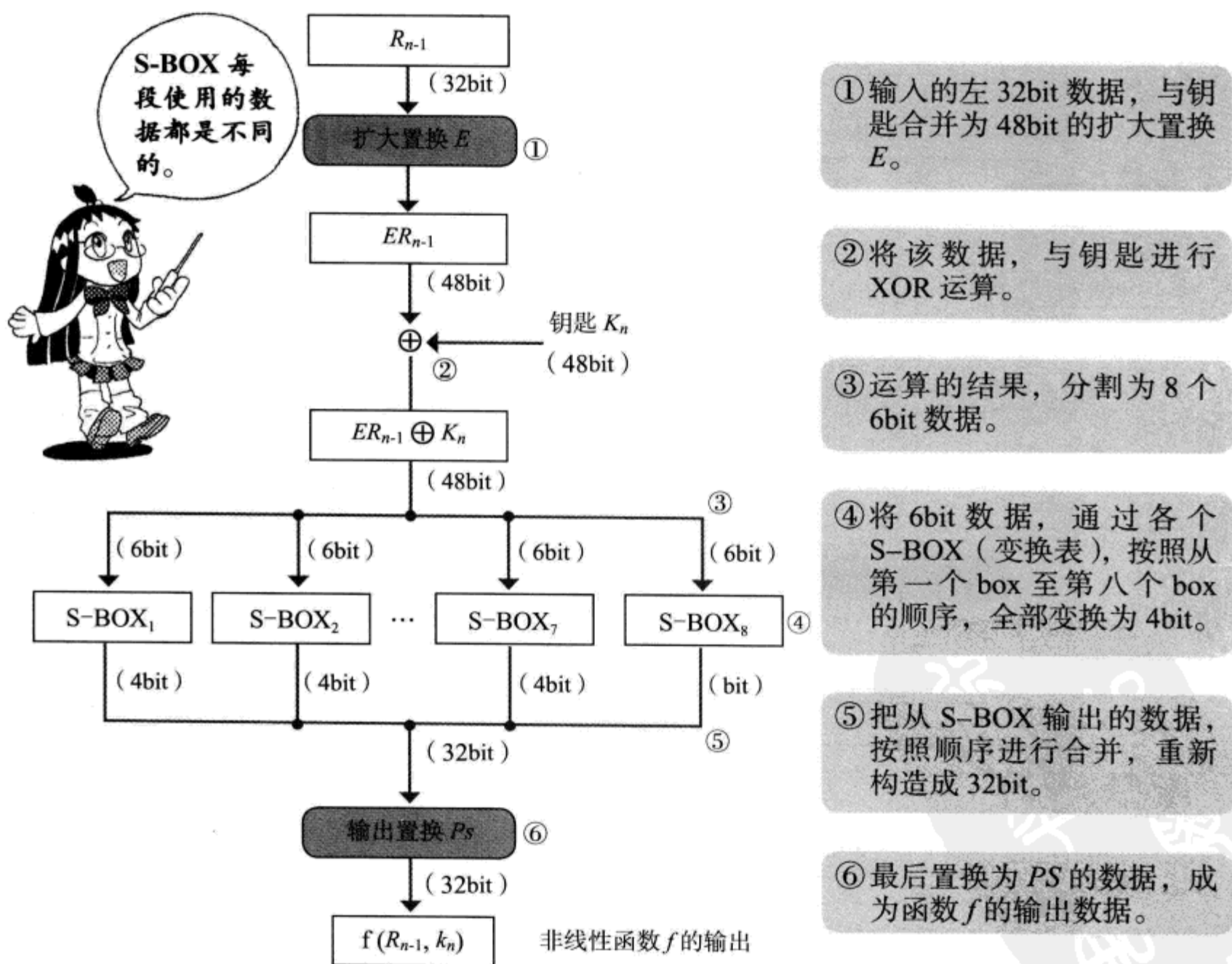
图 2.8 DES 的非线性函数 f 的构成
