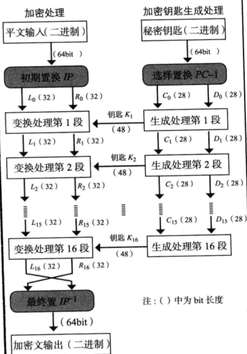
图 2.9 DES 加密的基本构成
