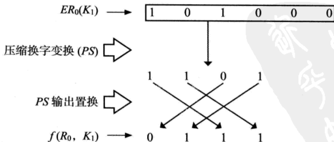
图 2.18 “步骤 5” 计算流程
