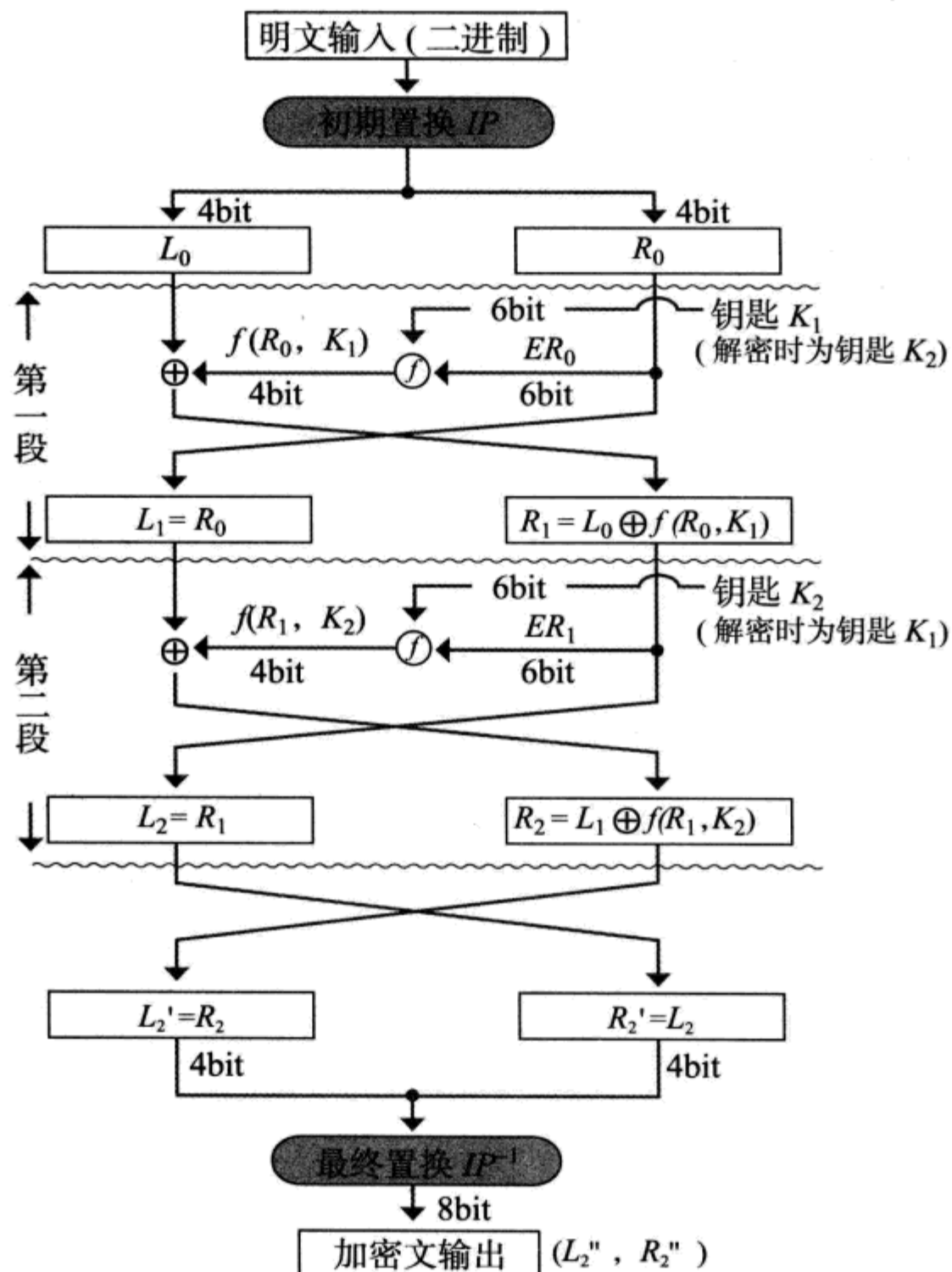
图 2.12 简易版 DES 加密文的生成顺序
