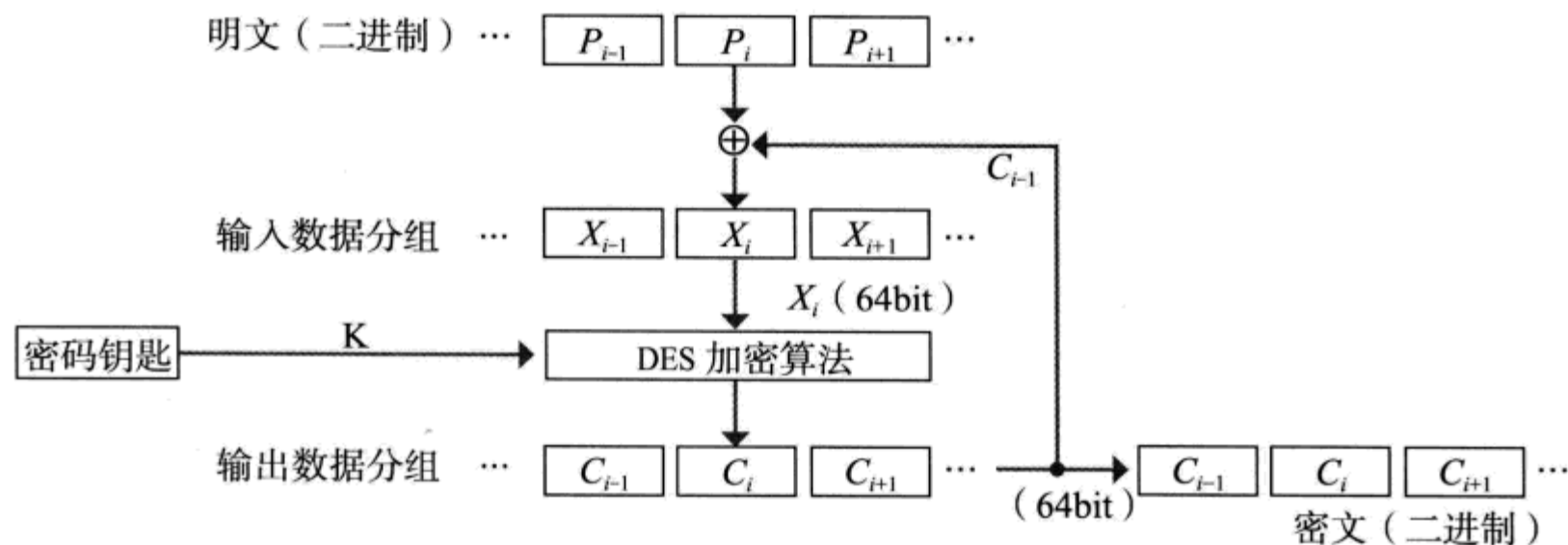
图 2.5 CBC 的结构
