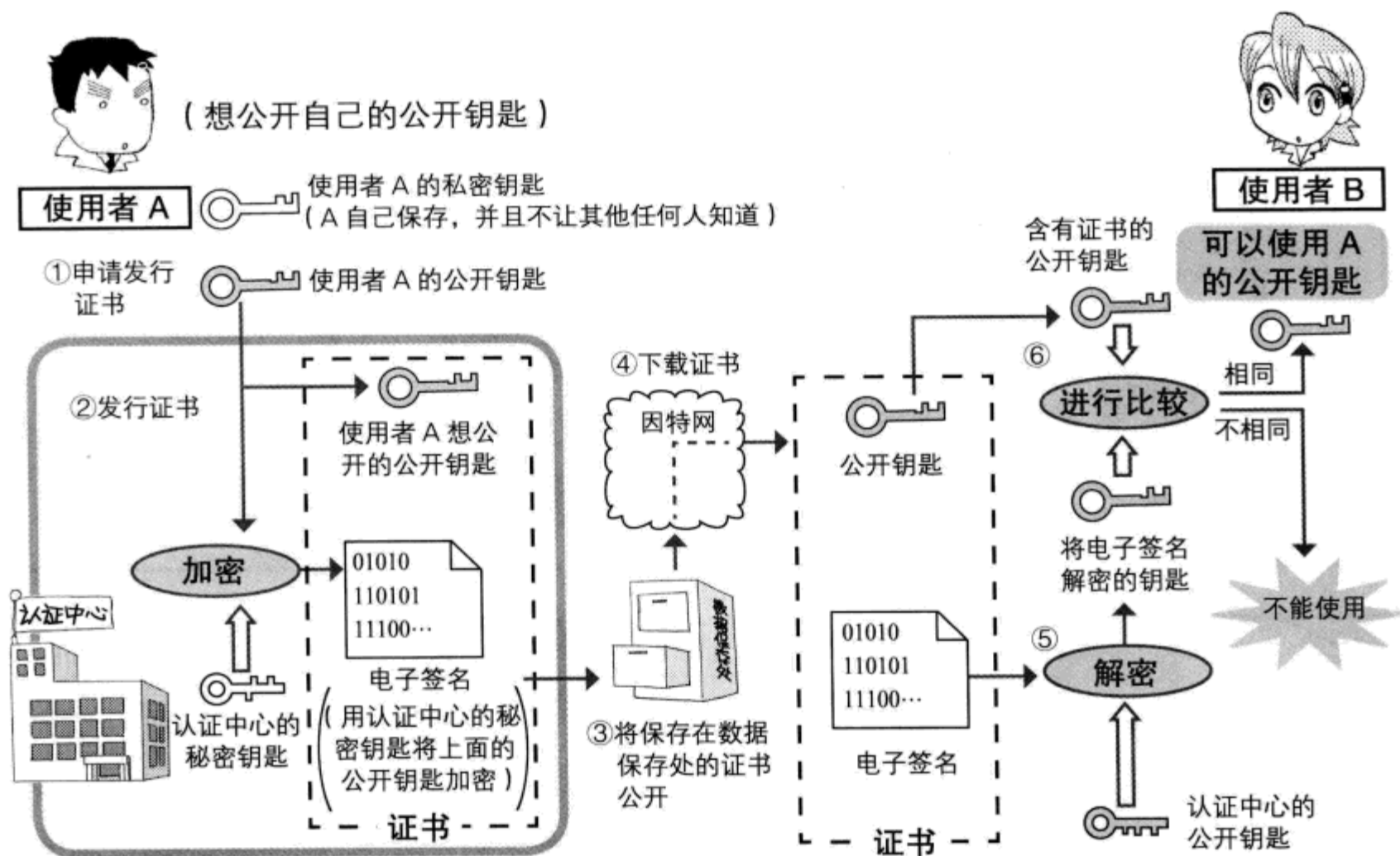
图 4.7 发行证书的流程
