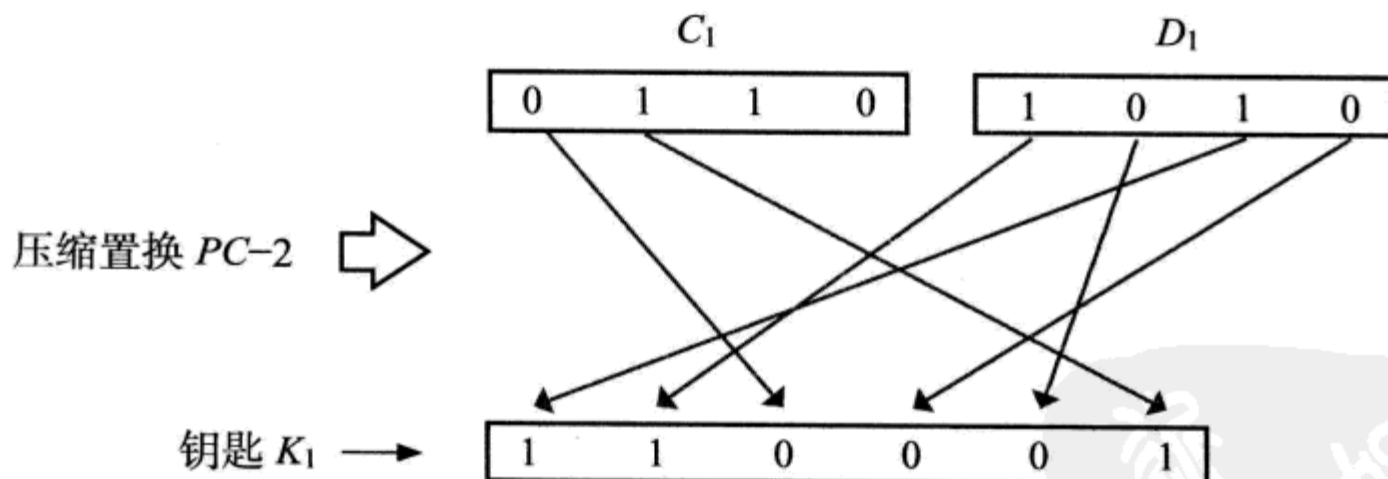
图 2.28 压缩置换 PC-2 的处理 “步骤 3”
