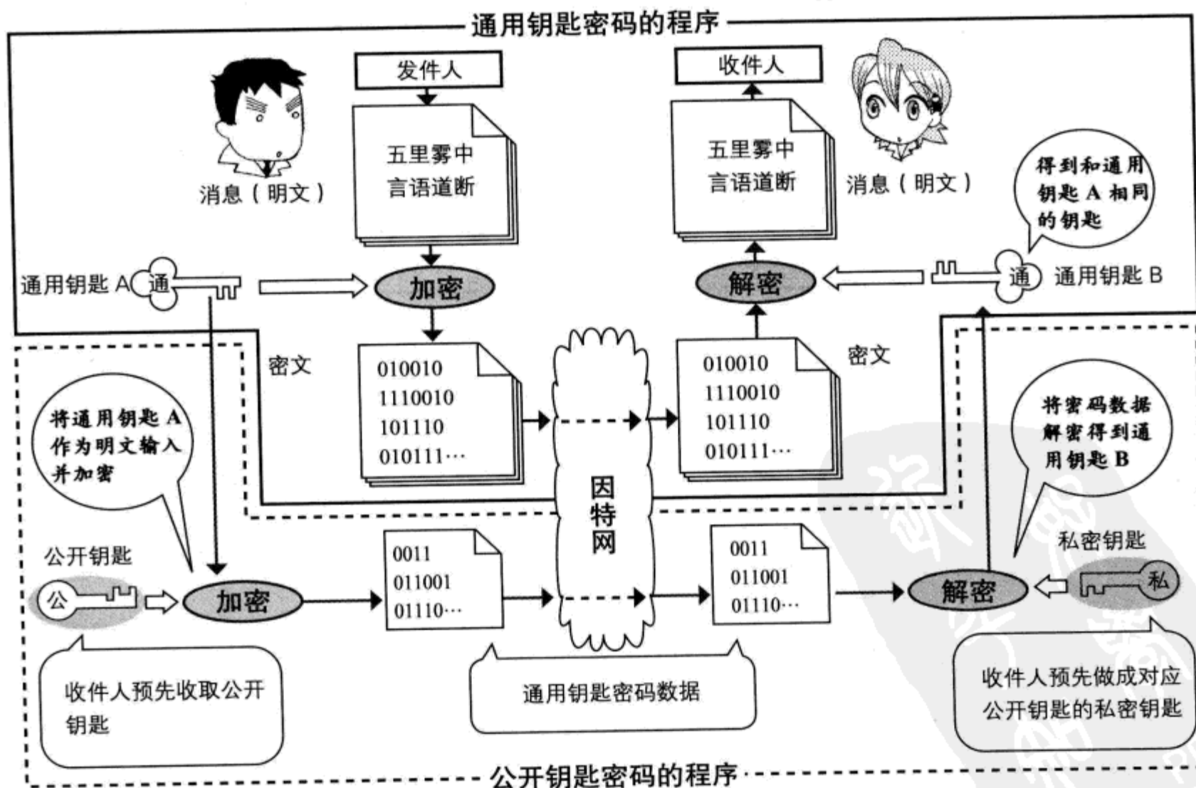
图 4.1 Hybrid 密码的加密和解密的流程
