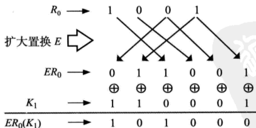
图 2.17 步骤 4 的计算流程
