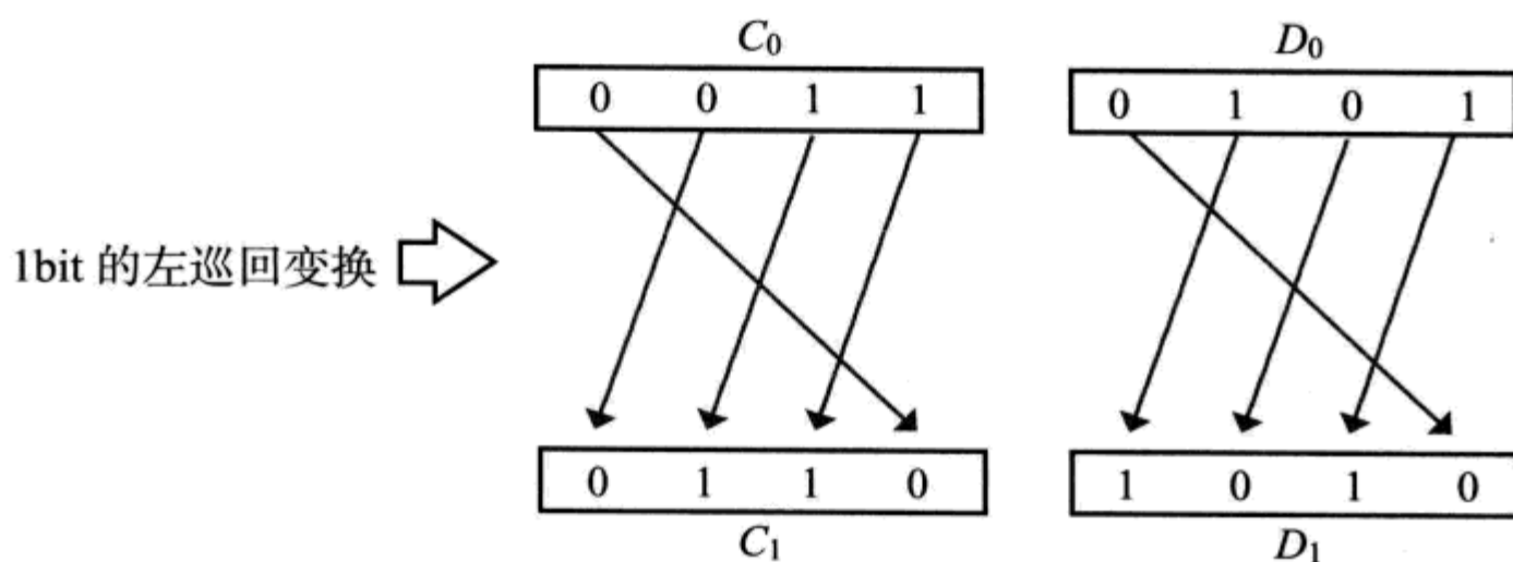
图 2.27 左巡回变换的处理 (步骤 2)
