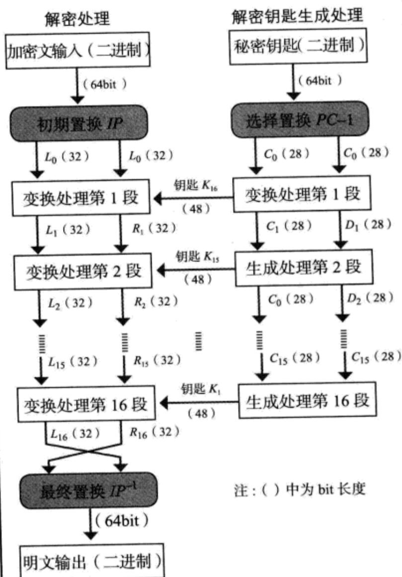
图 2.10 DES 解密的基本构成
