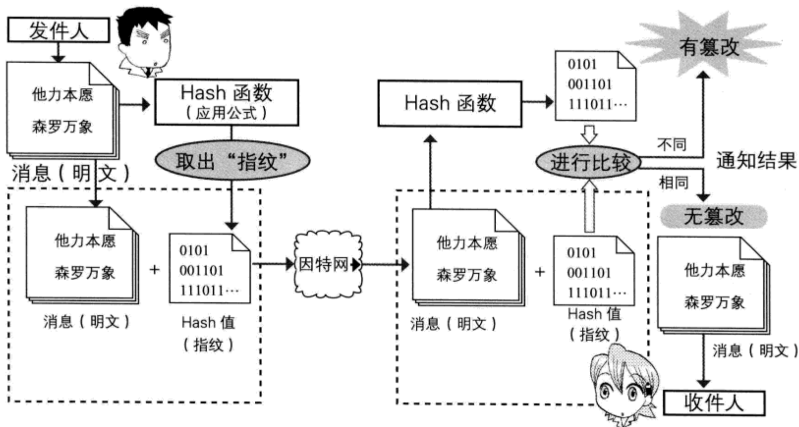
图 4.2 Hash 函数
