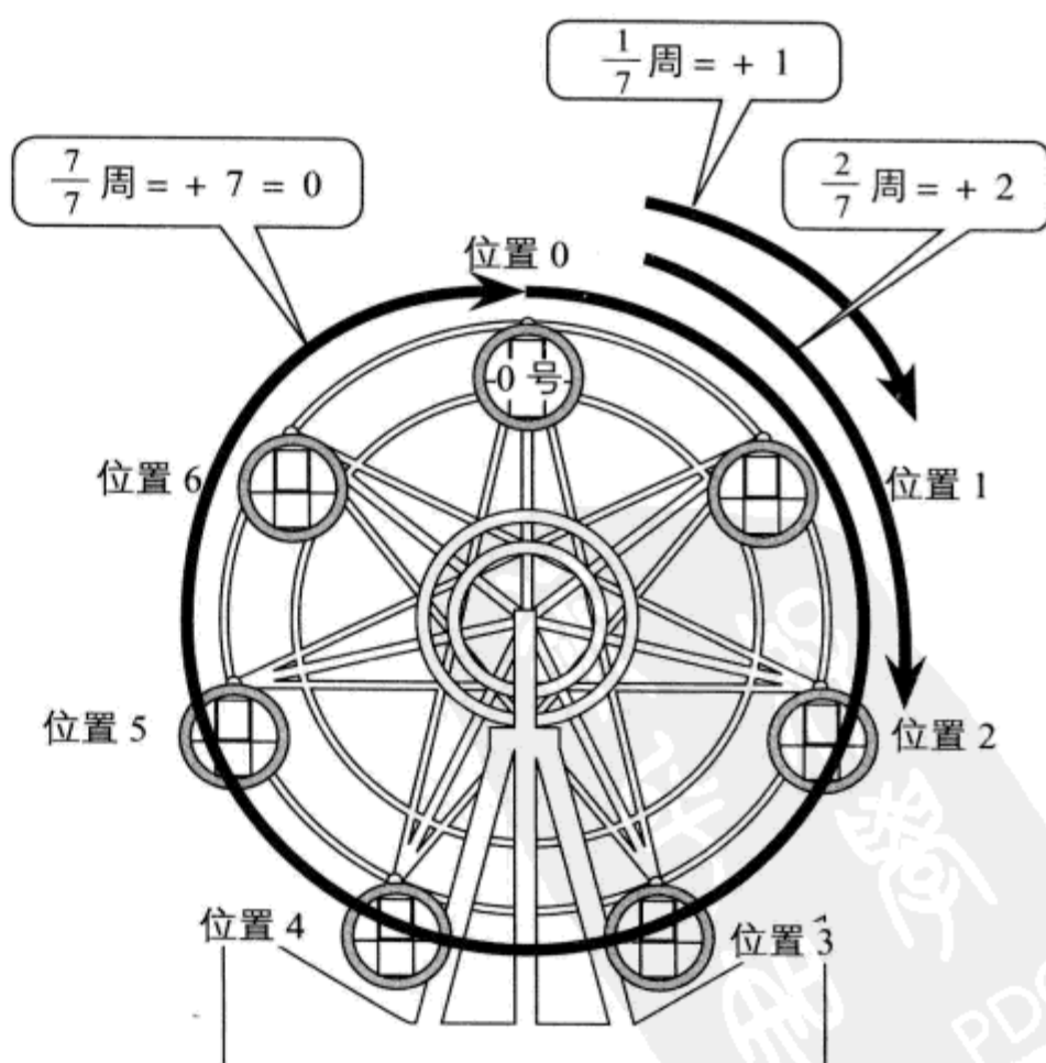
图3.2 取模加法运算的模型 (1)
