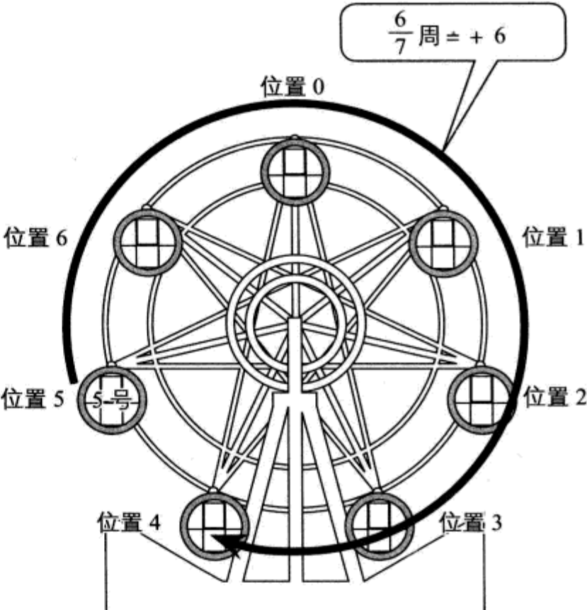
图 3.3 取模加法运算的模型 (2)
