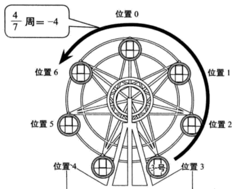
图 3.5 取模减法运算的模型 (2)
