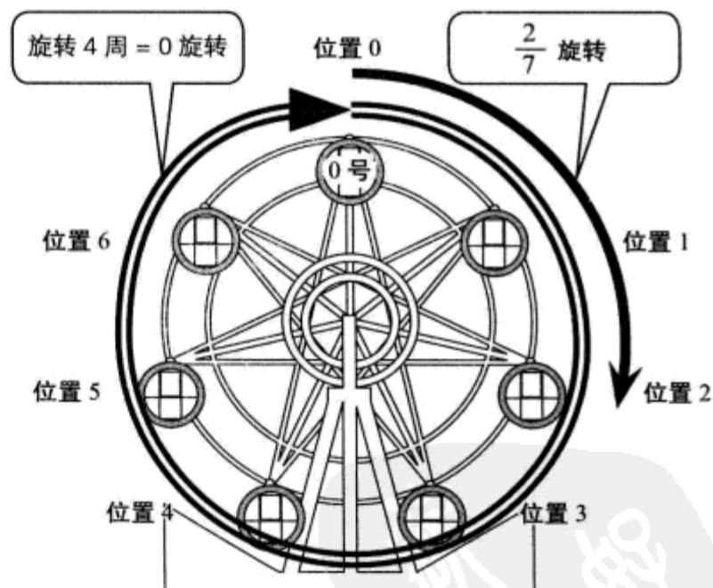
图 3.7 当 1 分钟旋转 \frac{5}{7} 周时, 6 分钟后的位置
