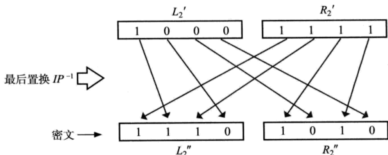
图 2.20 基于最后置换 IP^{-1} 输出的密文
