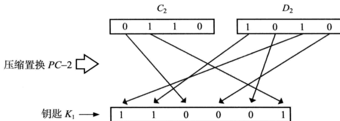
图 2.34 压缩置换 PC-2 的处理 “步骤 5”
