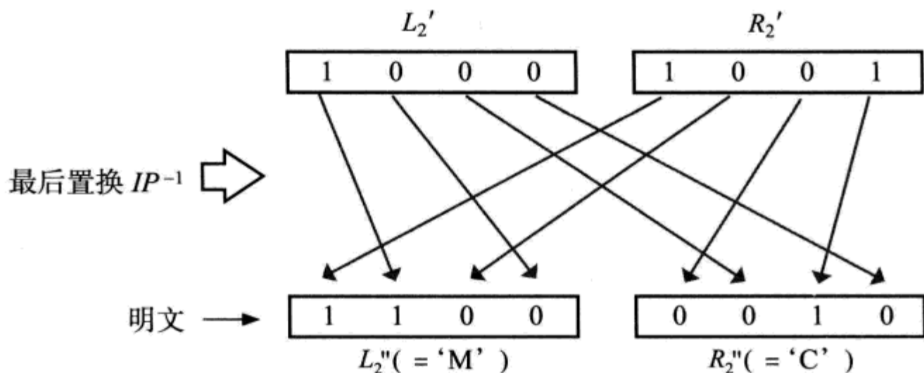
图 2.23 步骤 12 的计算流程
