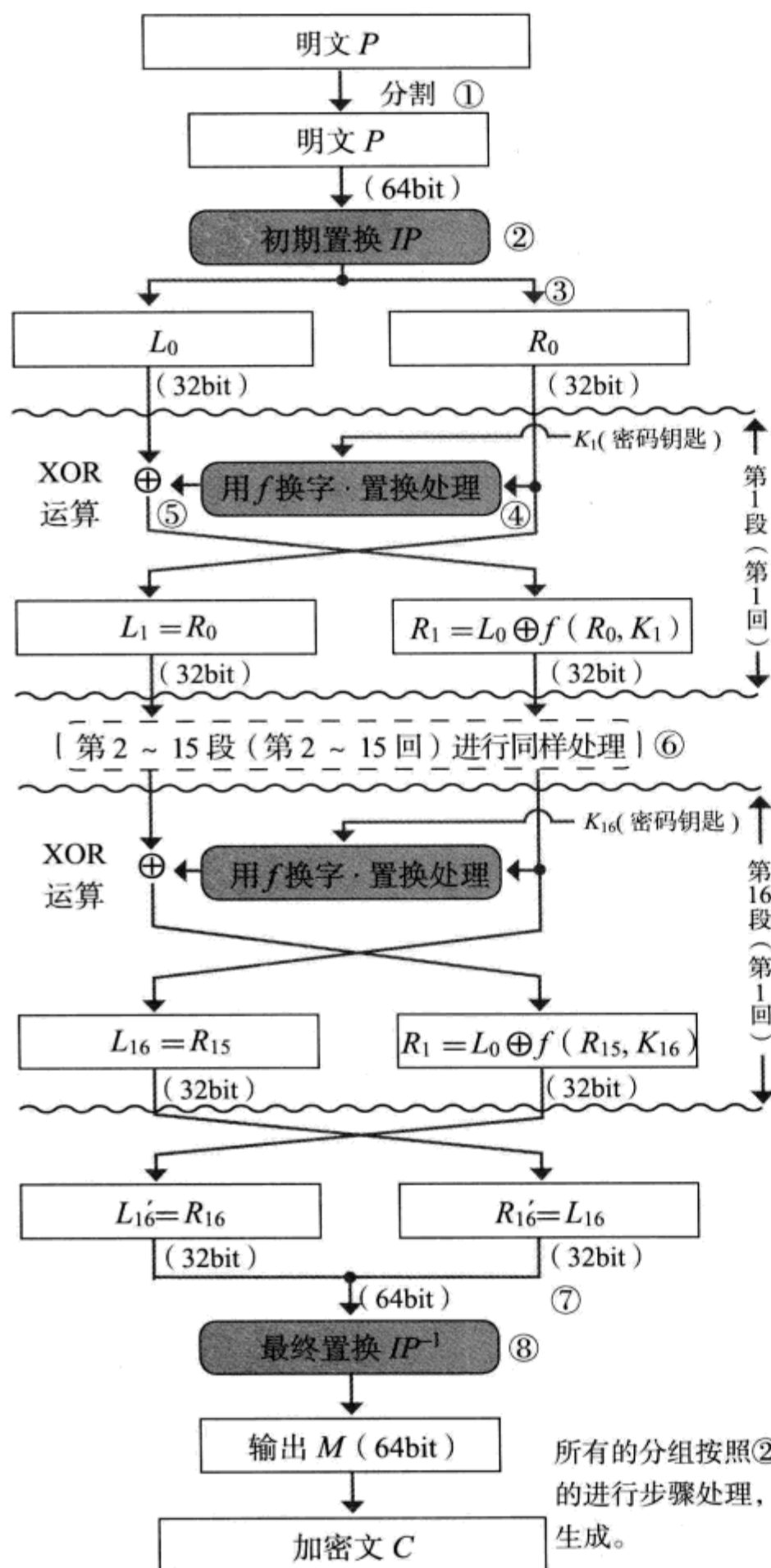
图 2.6 DES 加密顺序 (加密文的生成)
