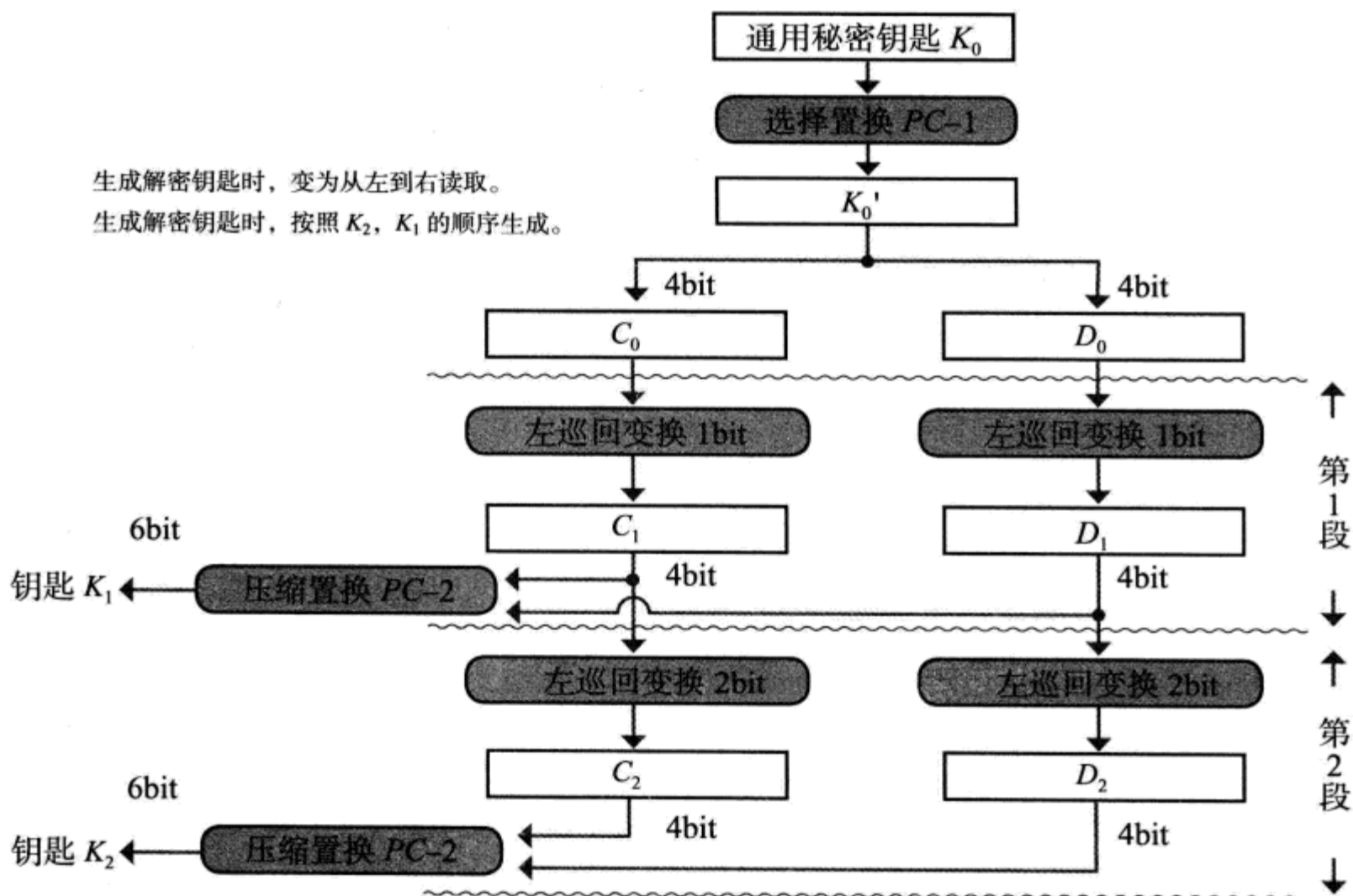
图 2.25 加密密钥和解密密钥的生成过程
