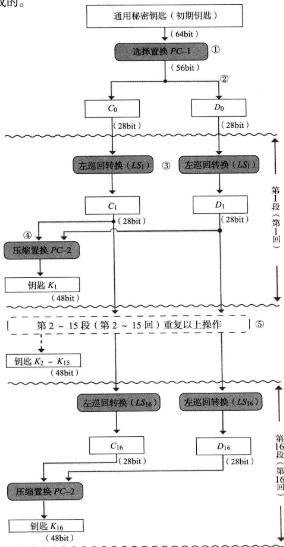
图 2.7 DES 密码的加密密钥和解密密钥的生成顺序
