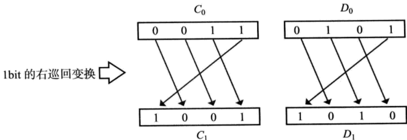
图 2.31 右巡回变换的处理 (步骤 2)
