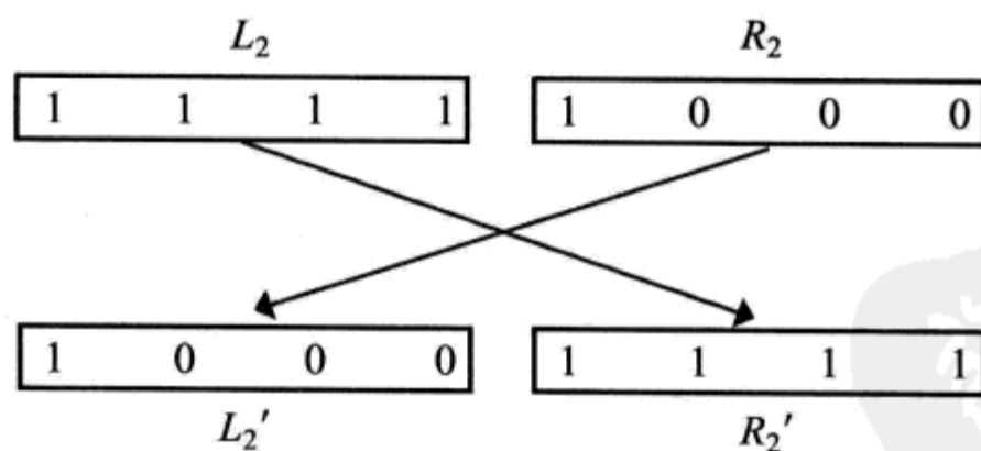
图 2.19 步骤 11 的计算流程
