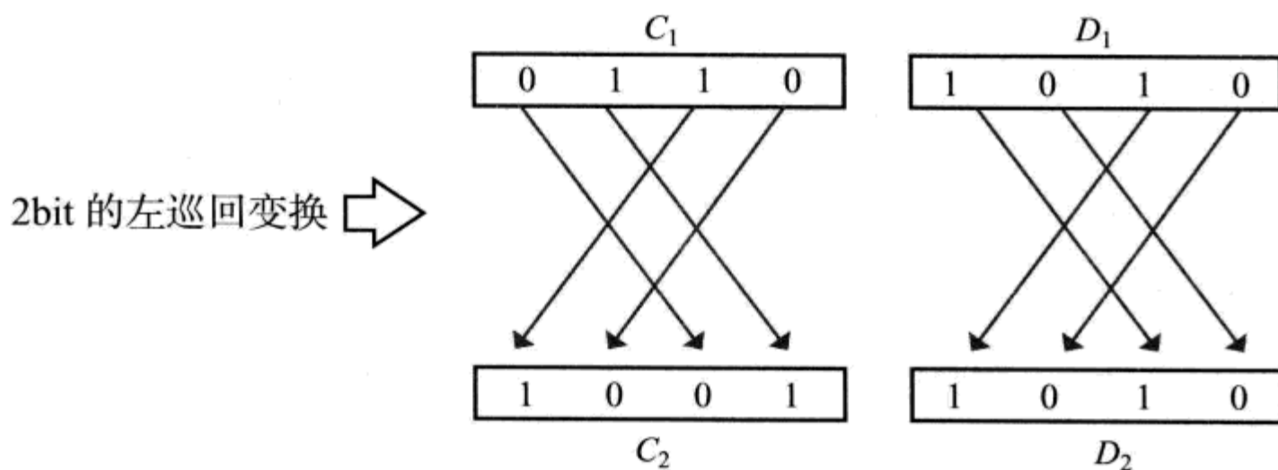
图 2.29 左巡回变换的处理 (步骤 4)
