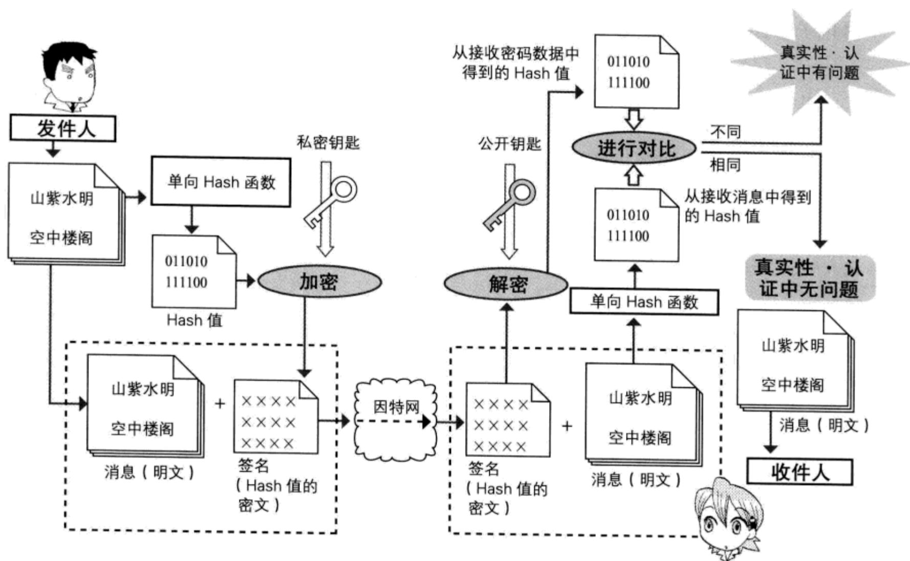
图 4.5 电子签名的构成 2 (将被 Hash 化的消息进行加密并署名的情况)
