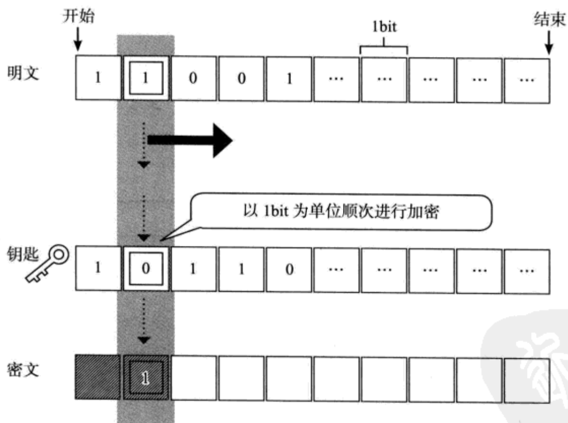
图 2.2 流密码的构成
