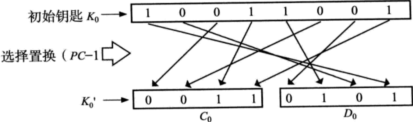
图 2.26 选择置换 PC-1
