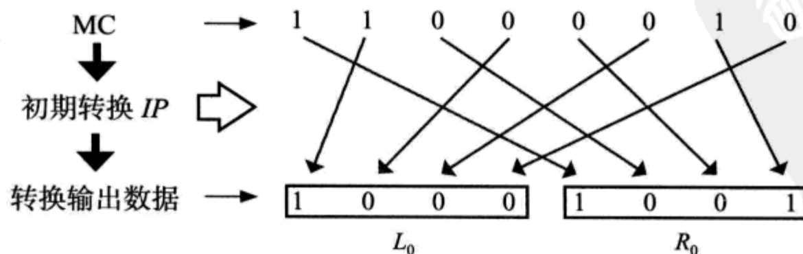
图 2.16 依据明文的初期转换 IP 输出数据
