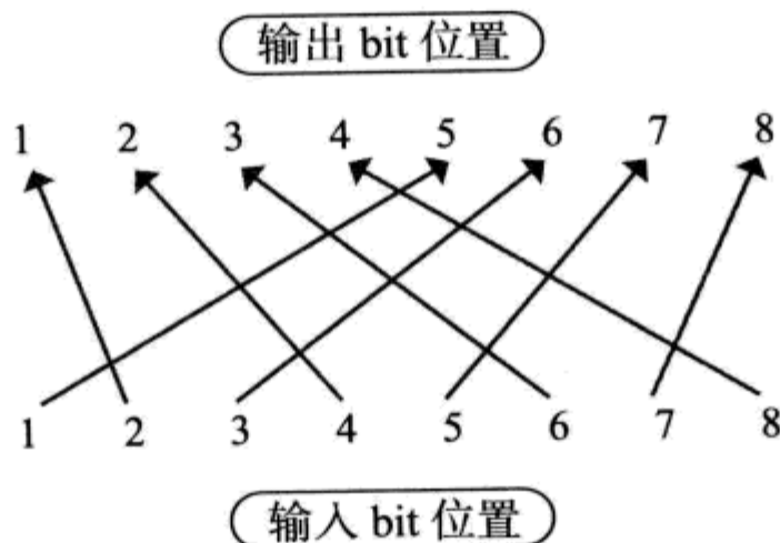
图 2.14 初期置换 IP 的另外一种表现
