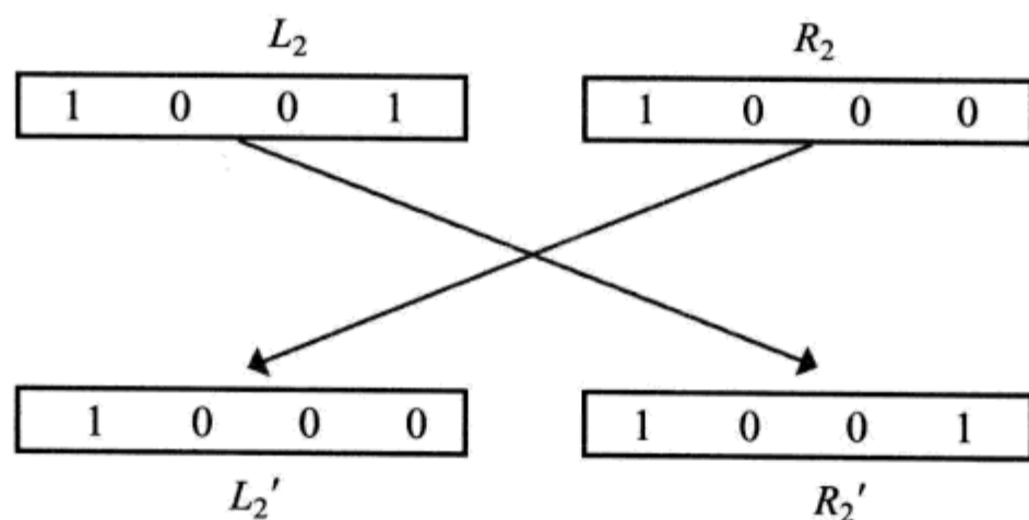
图 2.22 步骤 11 的计算流程
