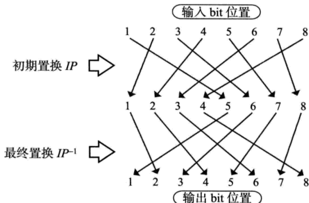
图 2.15 最初置换 IP 与最终置换 IP^{-1} 的组合
