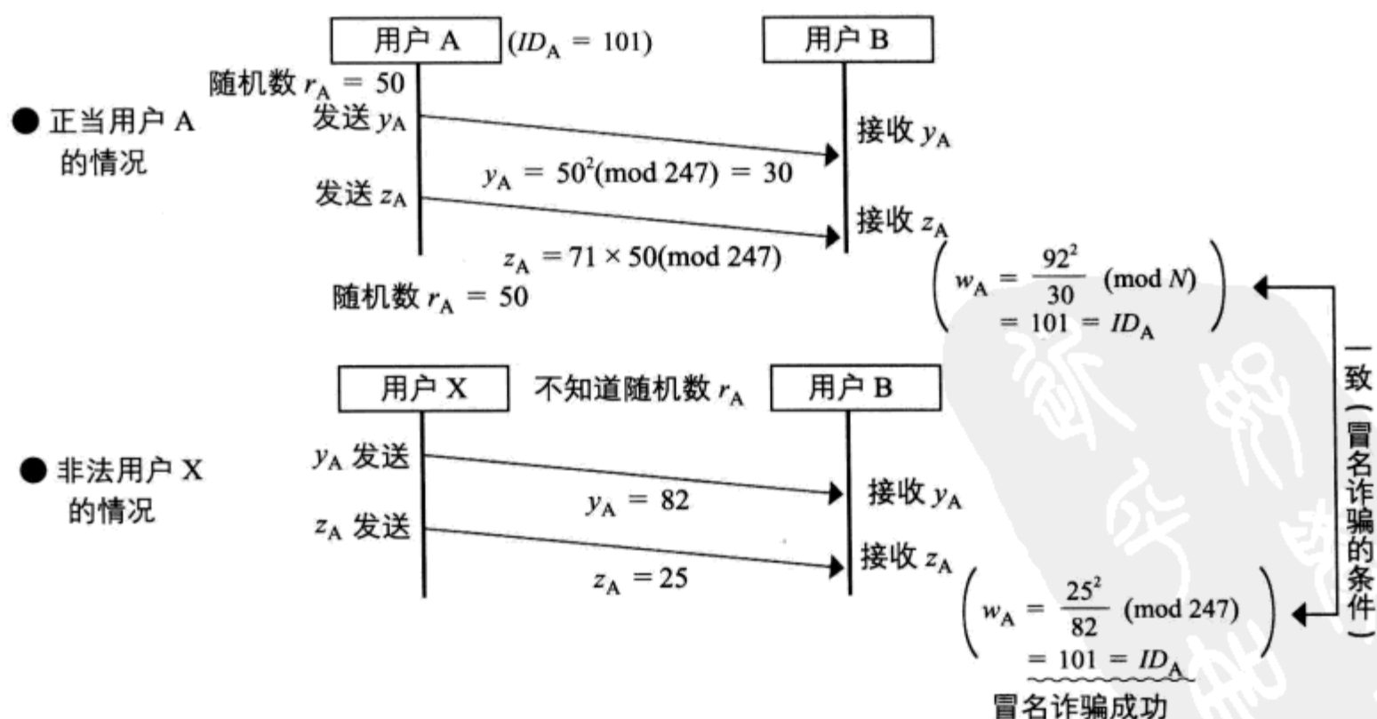
图 4.11 冒名诈骗的范例
