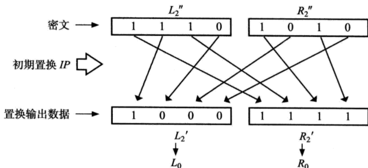
图 2.21 基于密文的初期置换 IP 输出数据
