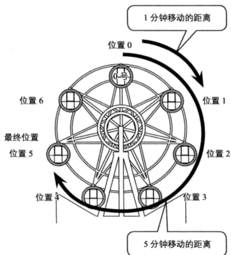
图 3.8 当 1 分钟旋转 \frac{1}{7} 周的状态 (2)
