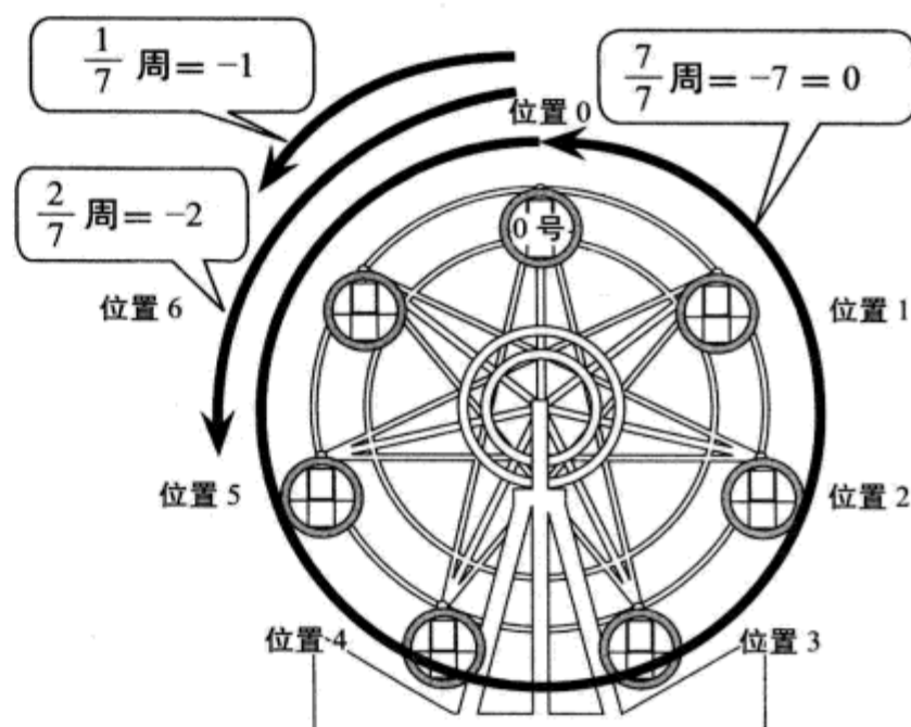
图 3.4 取模减法运算的模型 (1)
