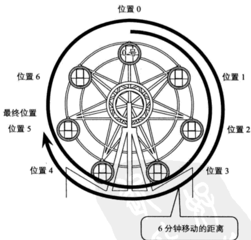
图 3.9 当 1 分钟旋转 \frac{2}{7} 周的状态
