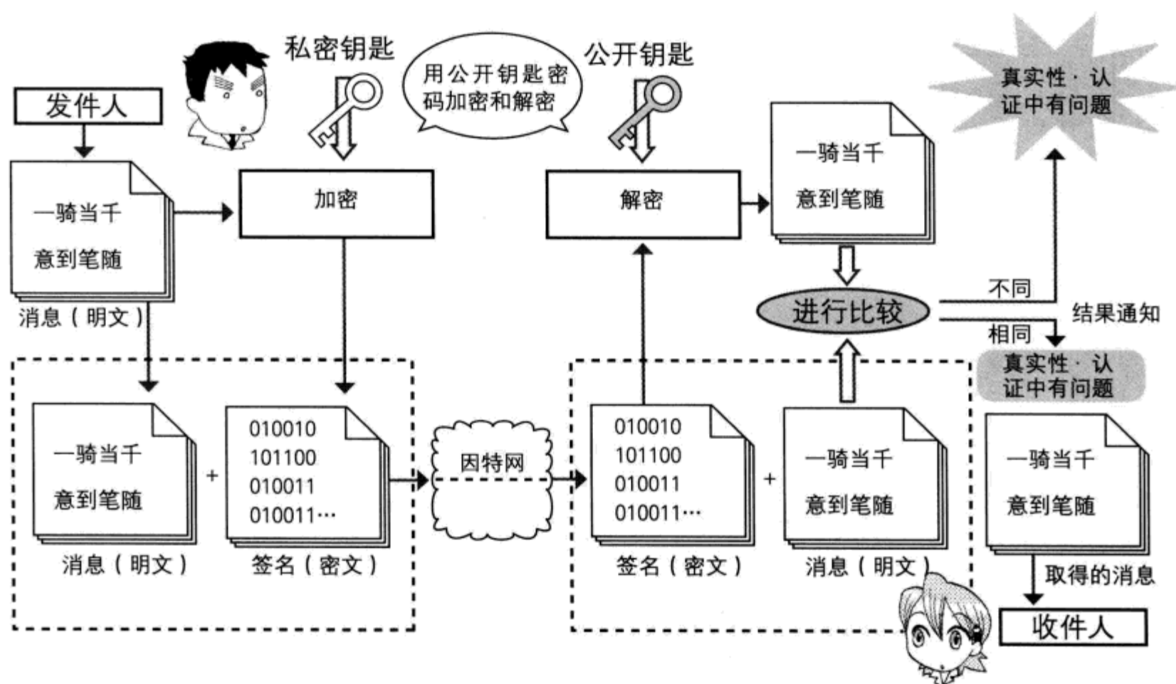
图 4.4 电子签名的构成 1 (将消息原本进行加密并签名的情况)
