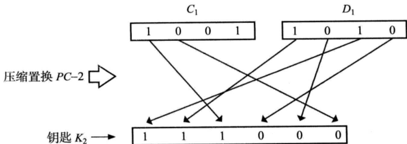
图 2.32 压缩置换 PC-2 的处理 “步骤 3”
