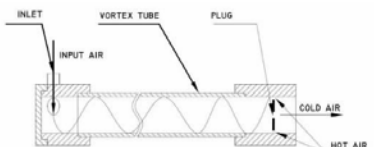
单孔设计的涡流管,左边注入压缩空气后,右边中央出冷气,外周出热气
