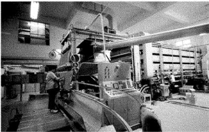
火柴杆通过这个机器后，就会附着上五颜六色的火药并进入传送带
