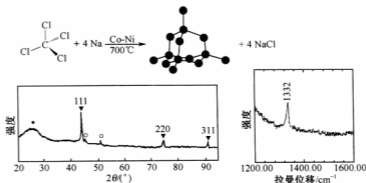
图1 所得产物的 XRD 和 Raman 光谱图
