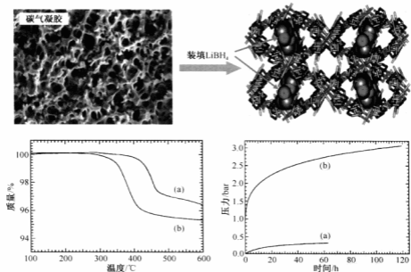
图1 \text{LiBH}_4 颗粒纳米化导致储氢性能改善
