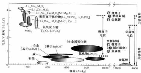
图2 锂二次电池正负极材料的电压和容量
