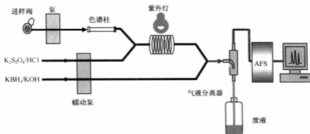
图1 用于汞形态分析的高效液相色谱与原子荧光光谱（HPLC-AFS）联用系统示意图
