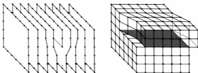
图2 边缘位错（左，红线标记）和螺旋（形）位错（右，切面标记）示意图
