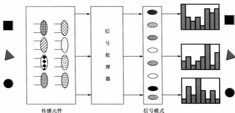
图1 仿生嗅觉和味觉传感器原理示意图
