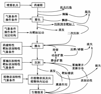
图1 农药喷雾时的剂量传递 [1]
