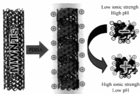
图1 聚二甲基二丙烯氯化铵非共价包覆的多壁碳纳米管用于分离酸性蛋白质的原理
