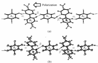
图 2 由 2, 5-dihydroxy-p-benzoquinone 和 5, 5'-dimethyl-2, 2'-bipy 形成的共晶在铁电相 [(a) 50K] 和顺电相 [(b) 293K] 的结构 293K 时无序的氢键形成中心对称的结构; 50K 时氢键有序化, 形成极化的结构 [8(a)]
