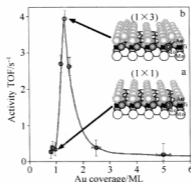
图 1 金纳米膜的一氧化碳催化氧化活性 (a) 单原子层金纳米膜, (b) 双原子层金纳米膜
