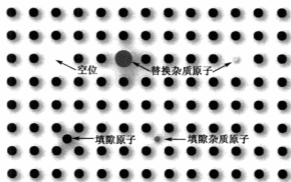
图1 点缺陷示意图
