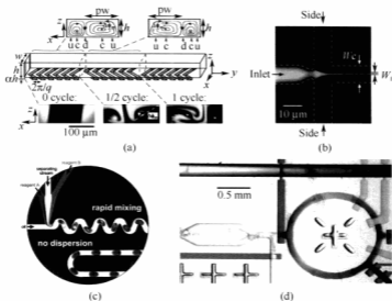
图1 几种常见的微流控混合装置
