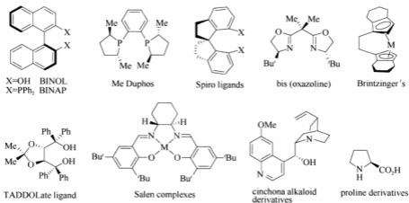
图 1 优势手性催化剂
