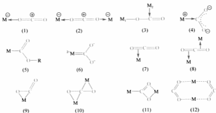
图2 活化二氧化碳的几种可能模式
