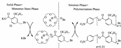
图2 非均相反应实现链式缩聚反应 [1]
