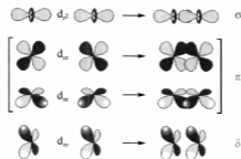
图 4 金属-金属键中的 \sigma 键、 \pi 键和 \delta 键 ( d_{z^2} 轨道主要形成金属-配体键)
