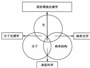
图1 包含光、分子和金属纳米结构相互作用的表面增强光谱学示意图
