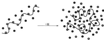
图 2 聚电解质构象变化
