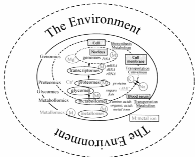
图1 金属组学研究 [2]
