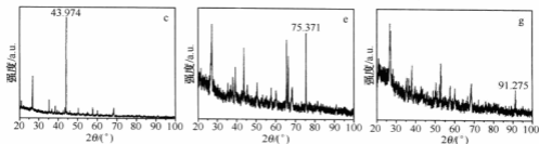
图 4 XRD 光谱图
