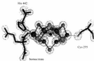
图 3 钼铁中心高分辨晶体结构图
