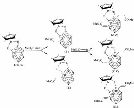
图1 碳硼烷分步定位取代
