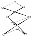
图 3 [\text{M}_2\text{Cl}_6]^{2-} 离子空间构型
