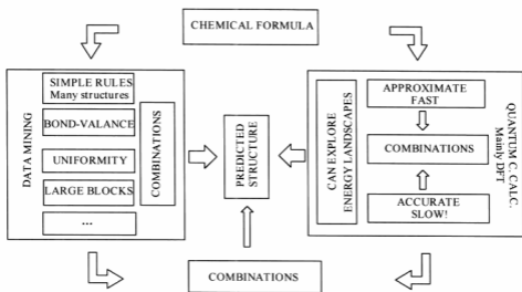
图1 结构预测路线图
