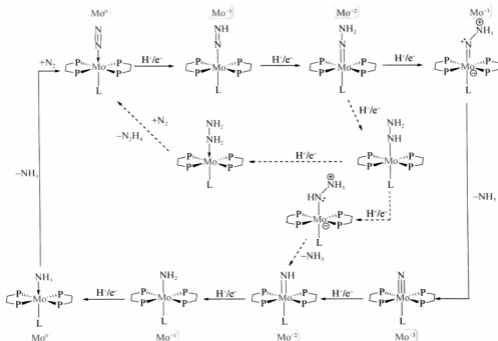
图 2 最初的 Chatt Cycle 示意图
