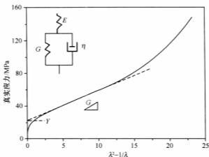
图 1 真实应力与应变关系及 Haward 模型示意图
