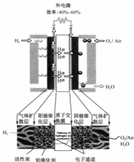
图 1 低温燃料电池的结构示意图
