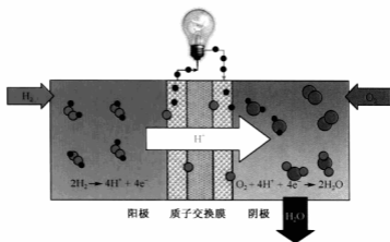
图 1 PEMFC 工作原理示意图
