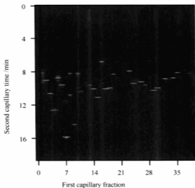
图1 二维毛细管电泳分离蛋白质酶解多肽图
