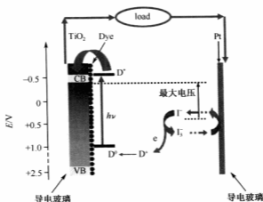
图 1 染料敏化太阳能电池结构示意图
