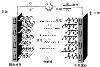
图1 锂离子电池工作原理示意
