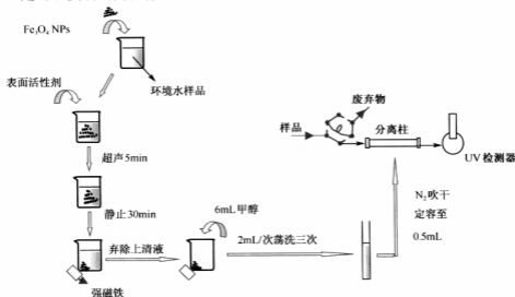
图1 纳米氧化铁固相萃取实验流程图
