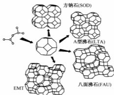
图 1 由方钠石笼组成的沸石结构
