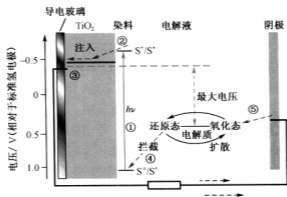
图1 DSSCs工作原理示意图
