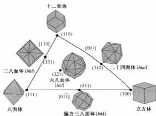
图2 面心立方金属单晶多面体三角形坐标系（单形赤平投影）
