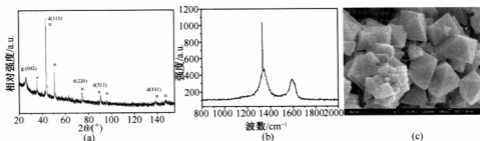
图2 所得产物的 XRD 光谱图 (a) (n-金刚石的衍射峰用“n”标出, 立方金刚石的衍射峰用“d”标出, 石墨的衍射峰用“g”标出)、Raman 光谱图 (b) 和产物的场发射扫描电镜图 (c)
