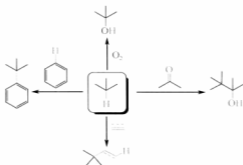
图1 新一代物质转化途径——C-H键活化
