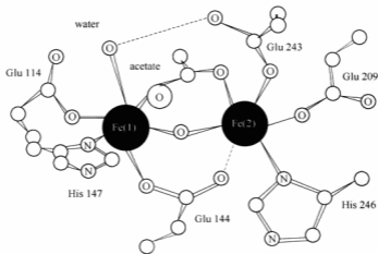
图 1 甲烷单加氧酶双核铁活性中心结构
