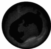
图 1 南极臭氧洞卫星观测图
