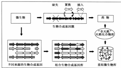
图1 组合生物合成的原理和方法
