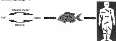
图1 汞的甲基化及其在生物体内的富集
