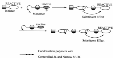
图1 取代基效应实现链式缩聚反应 [1]
