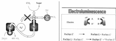
图1 植物光合作用中心 [8] 和电致发光材料与器件 [9] 的工作原理
