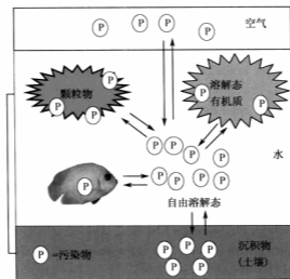
图1 环境中污染物的结合形态与生物有效性示意图
