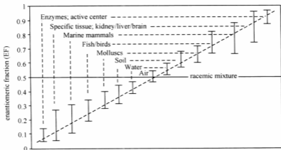
图 2 环境中手性化合物的 EF 值的偏离遵循原则
