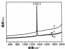
图 5 Raman 光谱图
