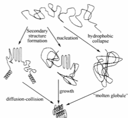
图2 蛋白质折叠微观理论模型 左边为骨架模型, 右边为疏水塌陷模型, 中间为成核-浓缩模型 [3]
