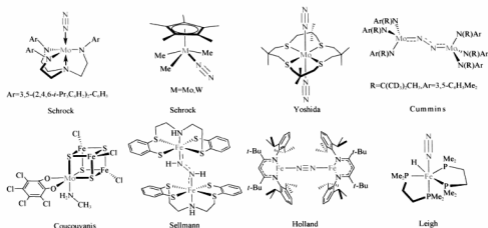
图4 活性固氮络合物
