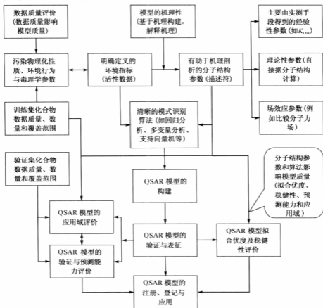
图1 基于机理分析而构建 QSAR 模型以及验证和表征 QSAR 模型的流程
