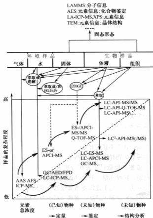
图 1 形态分析过程和方法 [4, 7]
