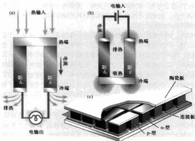
图1 热电材料温差发电、加电致冷示意
