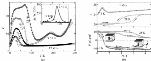
图 3 (a) \text{CdCr}_2\text{S}_4 的巨磁电容效应 [10] ; (b) \text{TbMn}_2\text{O}_5 中磁场引起的电极化翻转和电极化-磁场滞回行为 [11]
