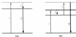
图 1 (a) 单光子激发发光过程：发射光 (3) 的光子能量小于激发光 (1) 的光子能量，通过与晶格作用，部分能量 (2) 转化为热能；(b) 双光子激发发光过程：发射光 (4) 的光子能量来源于过程 (1) 和 (3) 的两个光子能量，同时也有部分能量 (2) 转化为热能
