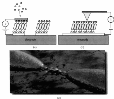
图1 电荷传输机理实验研究所采用的器件结构示意图
