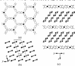
图 1 (BEDTTTF)_3[MnCr(C_2O_4)_3] 的晶体结构
