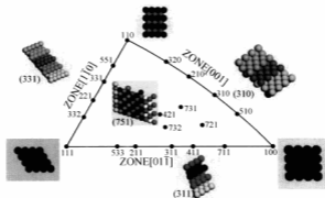
图1 面心立方金属单晶面三角形坐标系（单晶立体投影）
