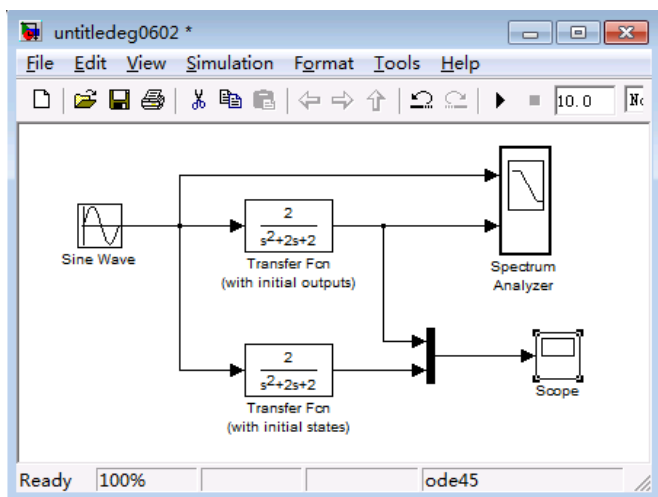
图 6-12 Simulink 模型
