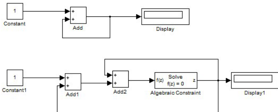
图 6-44 代数环样例
