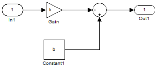
图 6-36 子系统中模块参数变量化
