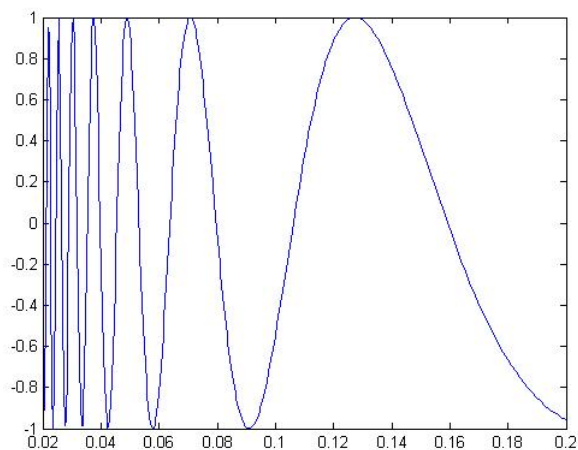
图 4-13 fplot 比较精确的图
