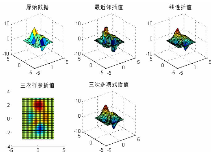
图 8-10 插值结果示意图
