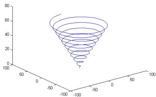
图 4-34 三度空间中的曲线
