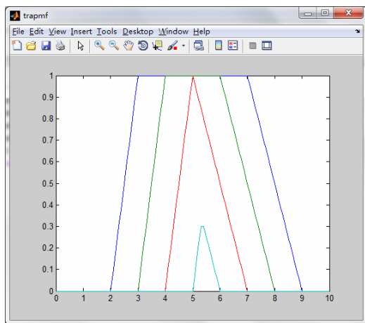
图 10-19 梯形隶属度函数曲线
