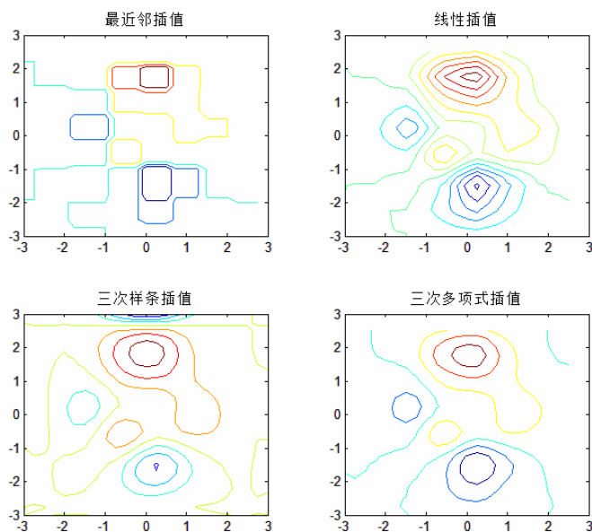
图 8-11 插值结果等高线示意图
