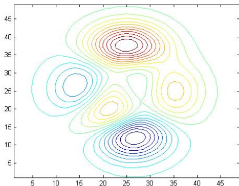
图 4-33 等高线在 XY 平面的投影
