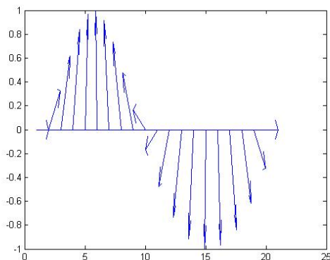
图 4-18 feather 函数举例 (2)
