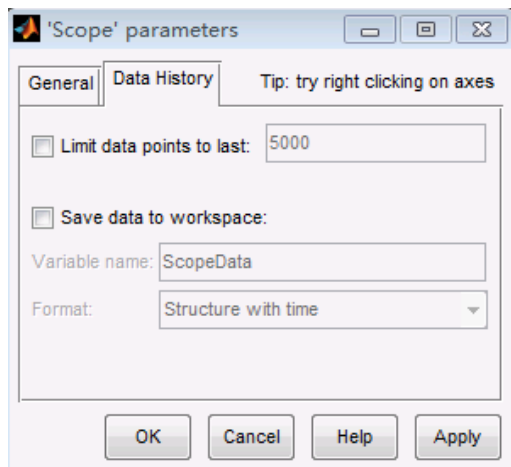
图 6-8 Scope 模块设置
