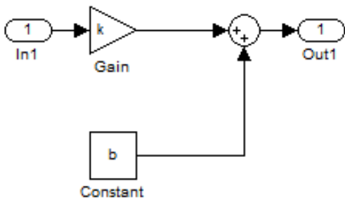
图 6-34 子系统模块内部结构图
