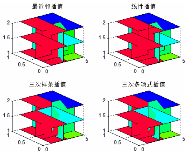
图 8-13 函数 flow 的三维差值结果
