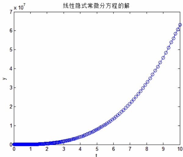
图 8-4 线性隐式常微分方程的解
