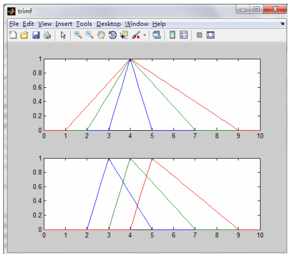
图 10-20 三角形隶属度函数曲线
