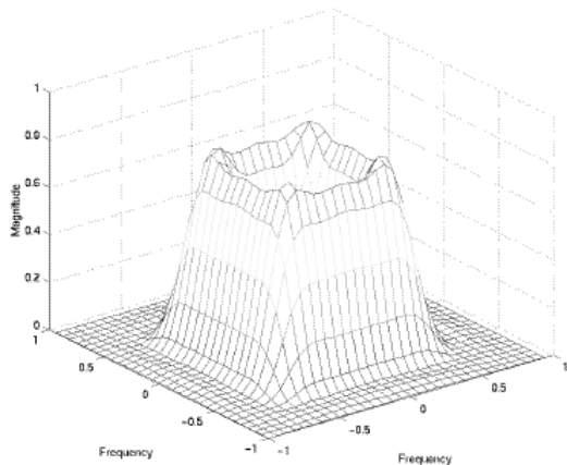
图 4-85 二维频率响应的计算
