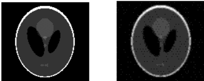
图 4-98 反 Radon 变换
