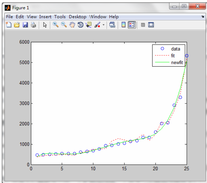
图 11-18 回归和曲线拟合结果显示
