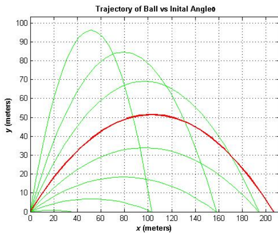
图 5-14 初始速度为 45 时的轨迹
