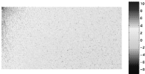
图 4-78 二维离散余弦变换
