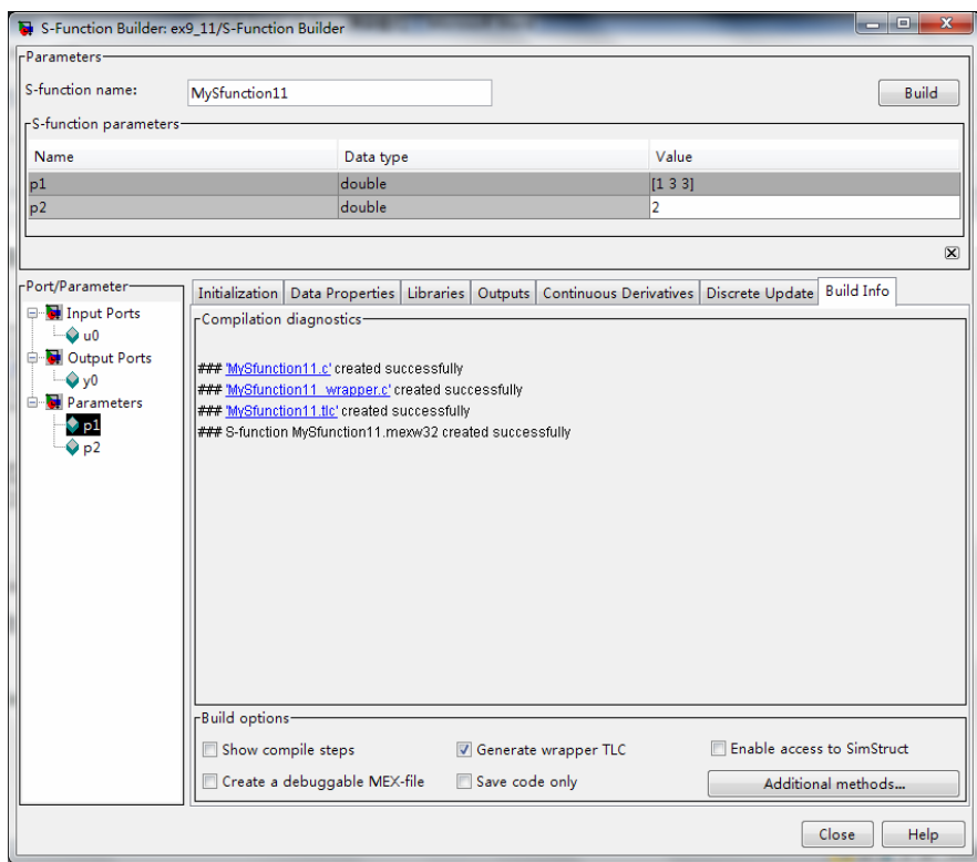
图 9-32 S-函数创建器编译结果
