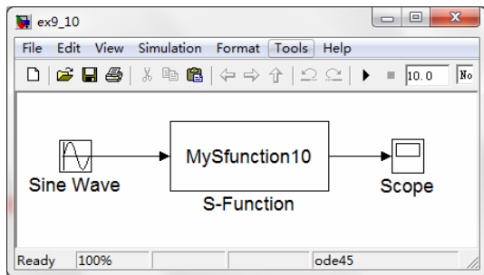
图 9-27 Simulink 仿真框图
