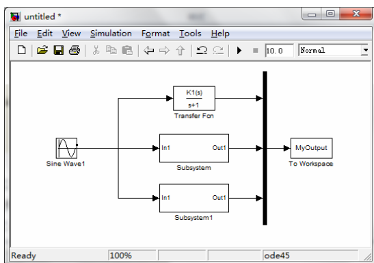
图 7-23 Simulink 模型
