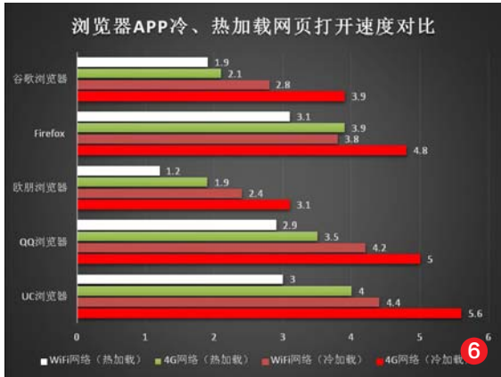
各大浏览器加载网页速度比较(单位:秒)
